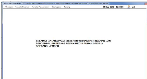
Gambar 4.9 Menu Utama
