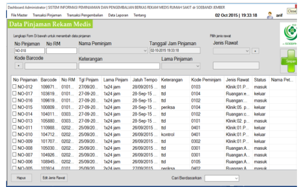
Gambar 4.10 Form Peminjaman
