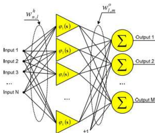
Gambar 2. RBF network dengan N inputs, L hidden units, dan M outputs [8]
